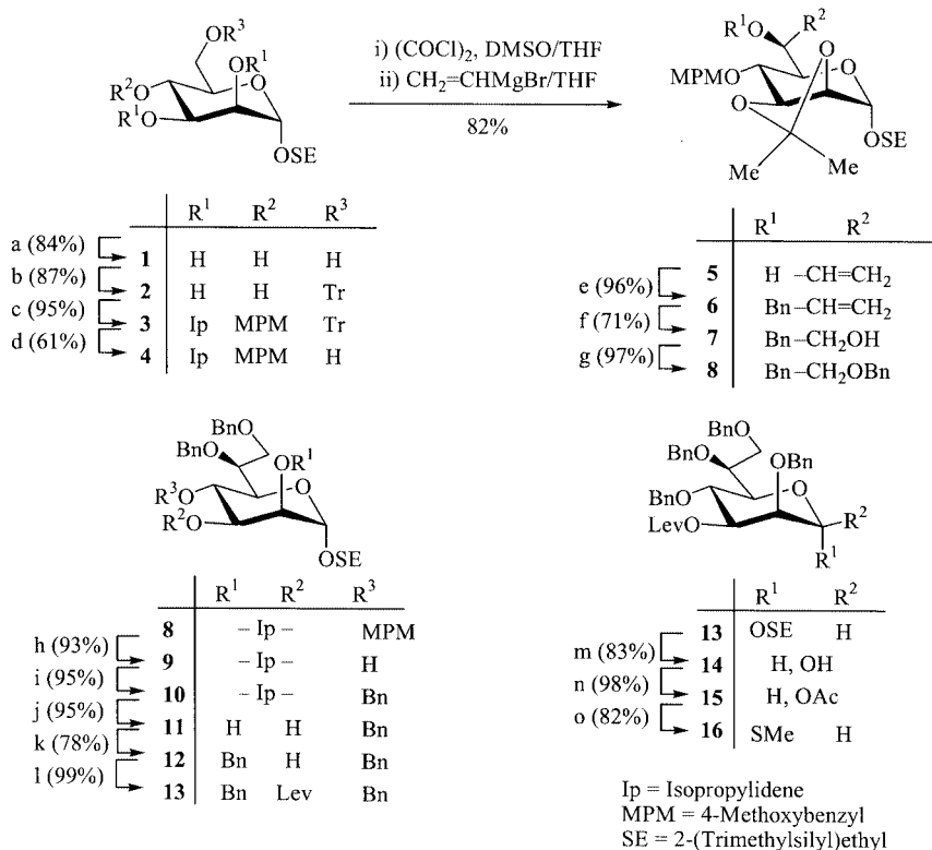
Scheme 1. Reagents: a) TrCl, DMAP/Pyr.; b) DMP, p -TsOH; c) MPMCl, NaH/DMF; d) AcOH; e) BnBr, NaH/DMF; f) (i) OsO 4 , NaIO 4 /tBuOH, (ii) NaBH 4 /CH 3 OH, H 2 O; g) BnBr, NaH/DMF; h) DDQ, H 2 O/CH 2 Cl 2 ; i) BnBr, NaH/DMF; j) 85% aq. AcOH; k) BnBr, TBAB/10% aq. NaOH, (CH 2 Cl 2 ); l) LevOH, DCC, DMAP/CH 2 Cl 2 ; m) TFA/CH 2 Cl 2 ; n) Ac 2 O/Pyr.; o) TMS-SMe, TMSOTf/CH 2 Cl 2
